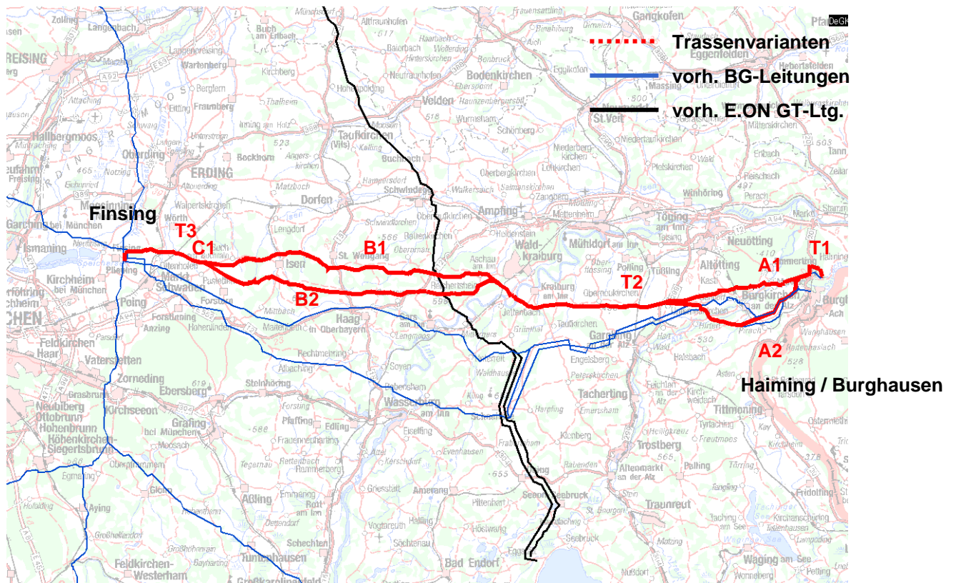
Abbildung 23: Übersicht der untersuchten Trassenabschnitte
